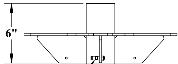
GROUNDING LUG
